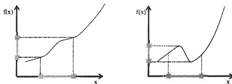
Slika 3: Grafička interpretacija propagacije neodređenosti pomoću intervalske matematike
