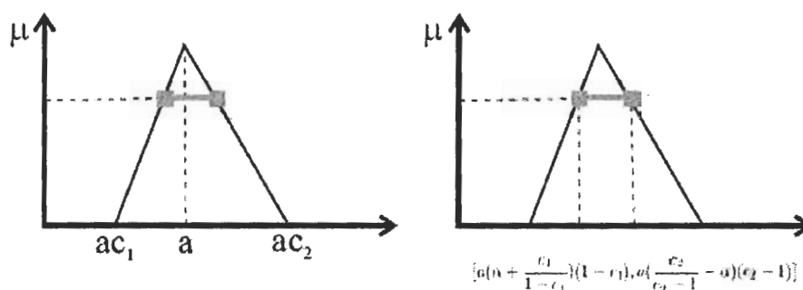
Slika 9: Parametri i \alpha presek trougaonog rasplinutog skupa
