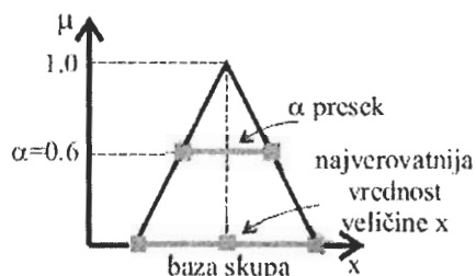
Slika 4: \alpha presek rasplintog skupa
