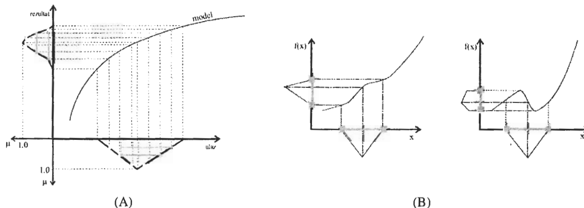
Slika 5: a presek metoda kod propagacije neodređenosti veličine u obliku rasplintog skupa
