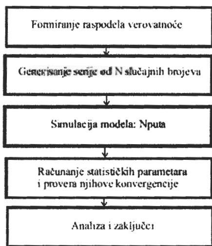
Slika 7: Procedura Monte Karlo metode
